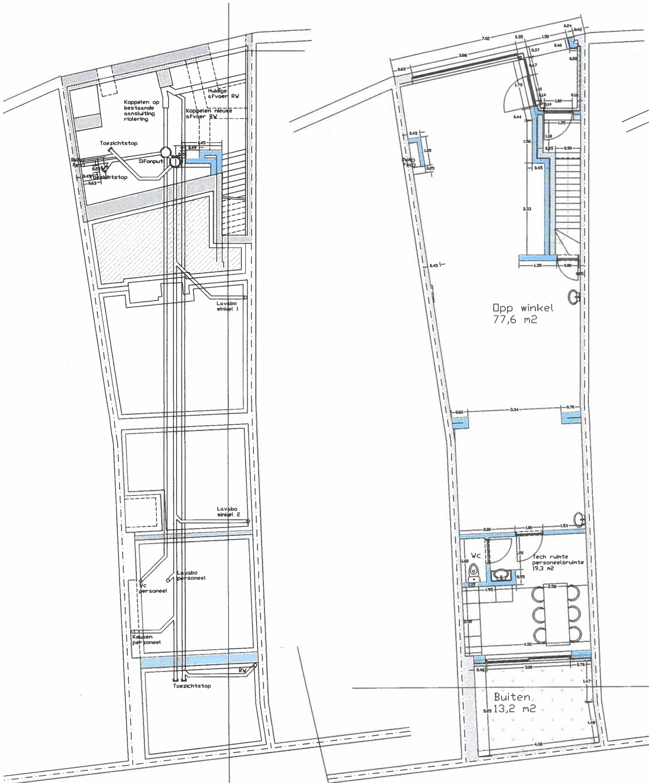
KELDER - FUNDERING + RIOLERING GRONDPLAN GELIJKVLOERS
